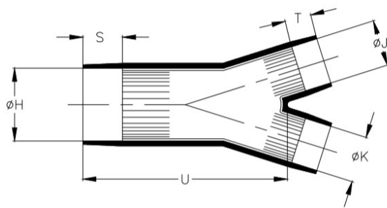
Vor Schrumpfung
